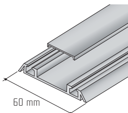
Profil S06NN krycí profil S06N
