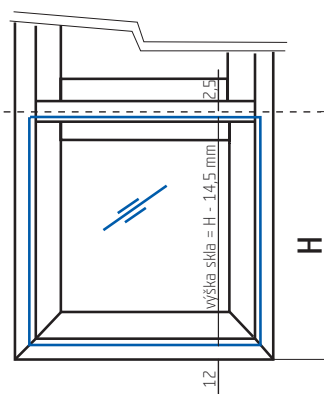
Příčka D:
