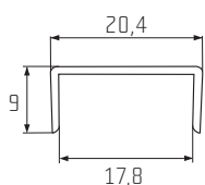
Profil U pro tl. desky 18 mm
