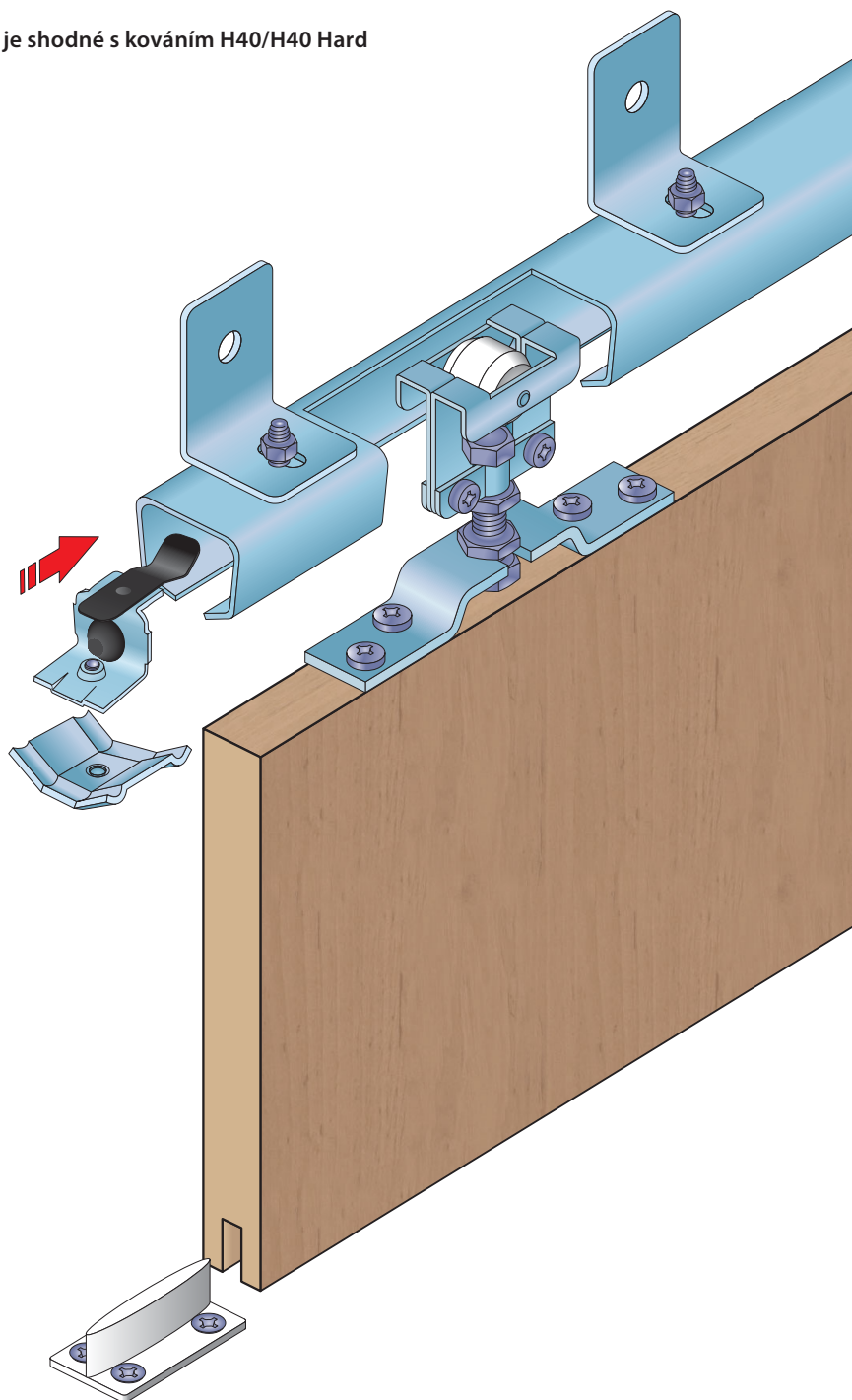
Sada S40H
