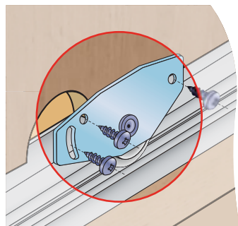
Montáž spodního jezdcce
