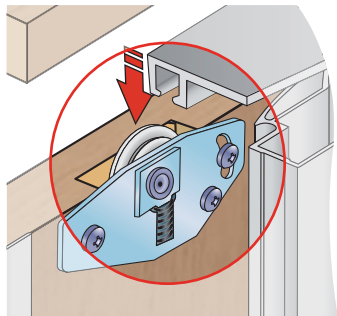
Montáž horního jezdcce
