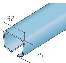
Horní ocelový profil S40/S80
