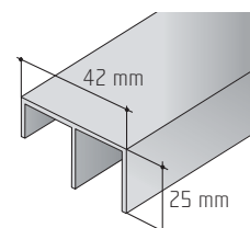
Dolní vodící profil S30
