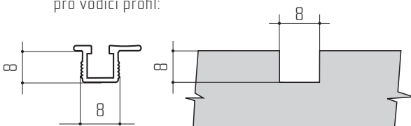
Vodící profil S03 (elox, délky 1,25; 2; 2,5; 3; 6 m)
