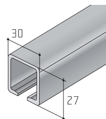
Horní hliníkový profil S40/S80
