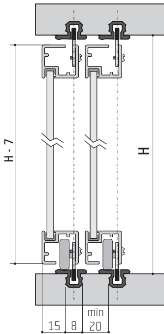
Horní vodítko
