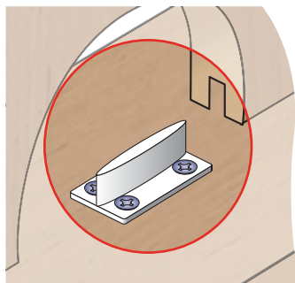
Montáž spodního kluzáku
