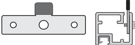
Jezdec s ložiskovým kolečkem a výškovou regulací
