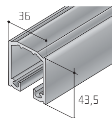
Profil S100
