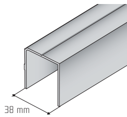
Profil S05-1
