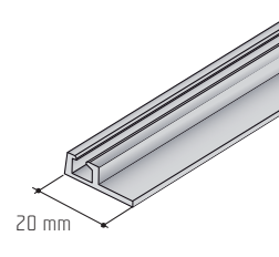
Profil S06N-1
