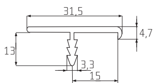
Narážecí hrana pro tl. desky 38 mm
