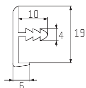
Narážecí hrana s madlem 02
