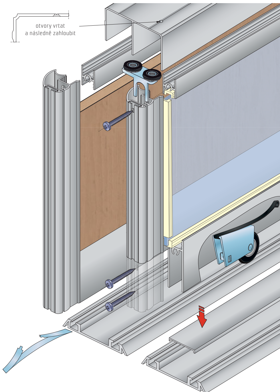
Profil S06NN krycí profil S06N
