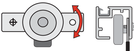
Jezdec s ložiskovým kolečkem a výškovou regulací
